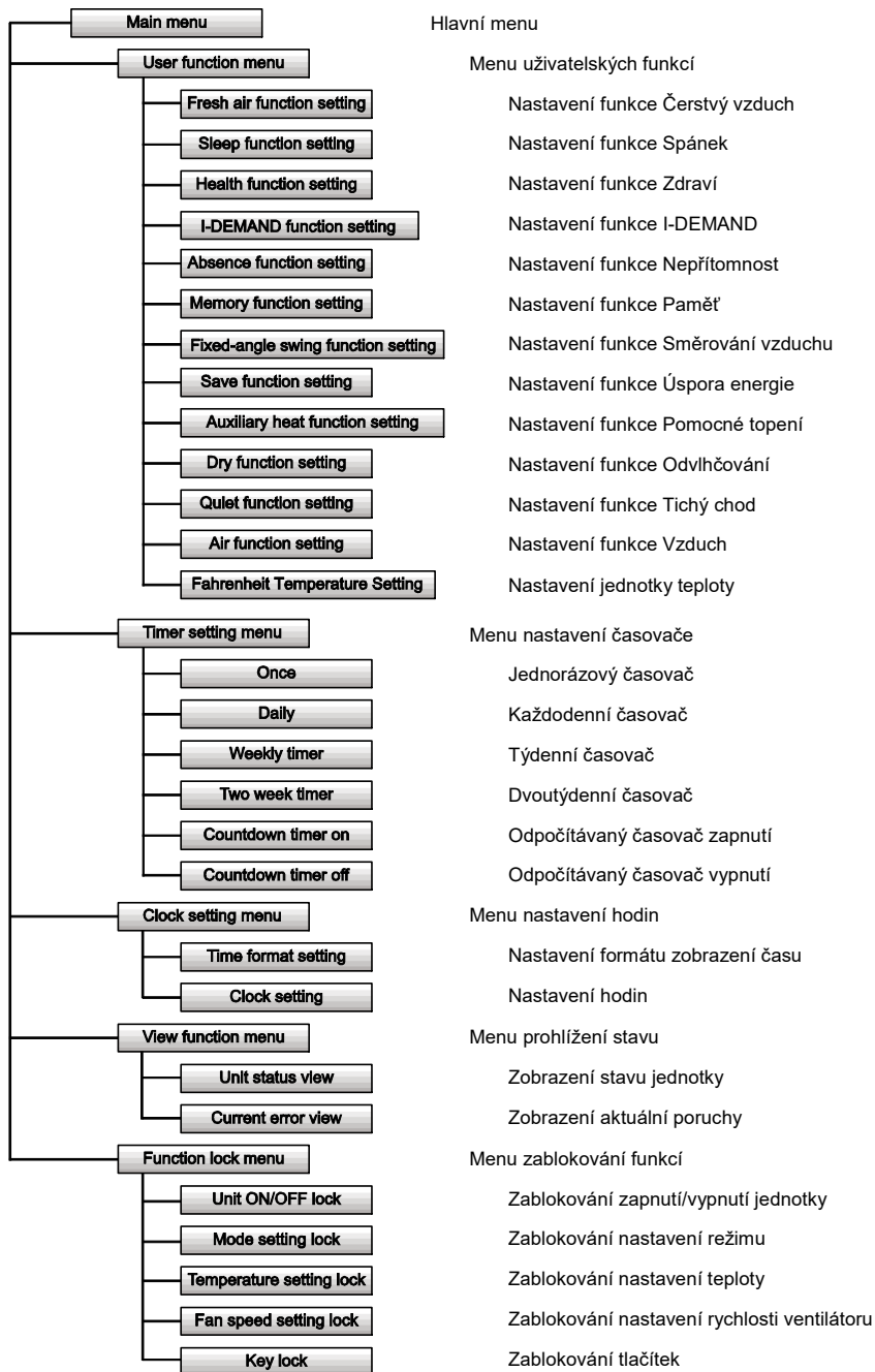
Obr. 3: Struktura menu
