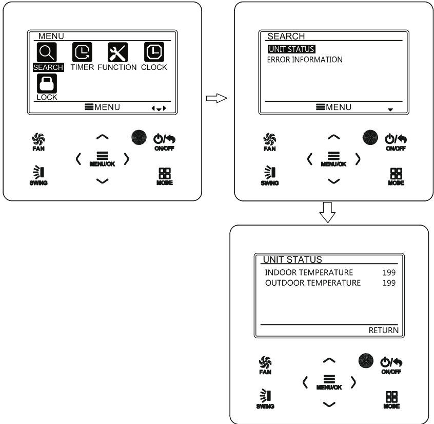
Obr. 9: Zobrazení stavu
