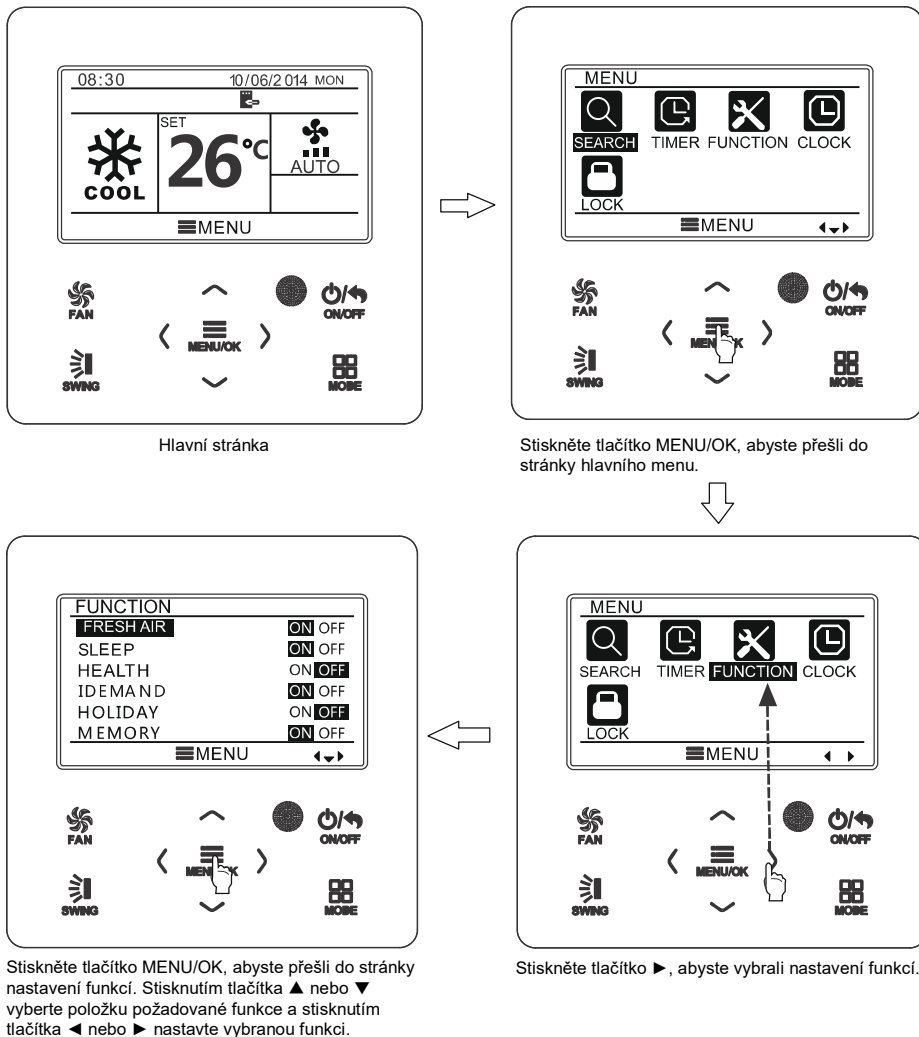
Obr. 8: Nastavení funkce
