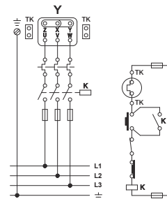
připojení ventilátoru k síti 3x400V
