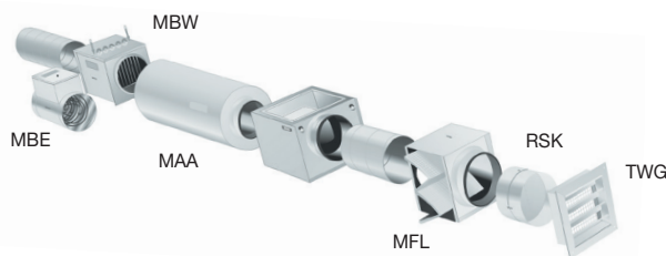
přívodní sestava
