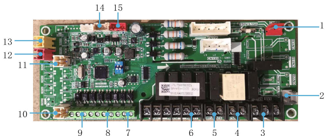
Obr. 8-10: Pomocná deska SCV-750EBH a SCV-1400EBH
