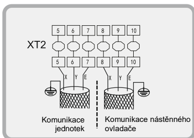
Obr. 8-18: Zapojení komunikace jednotek a komunikace nástěnného ovladače
