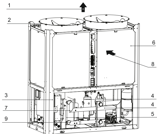
Obr. 8-3: Hlavní části SCV-1400EBH (Obrázek slouží jen pro zobrazení relativní pozice klíčových součástí)
