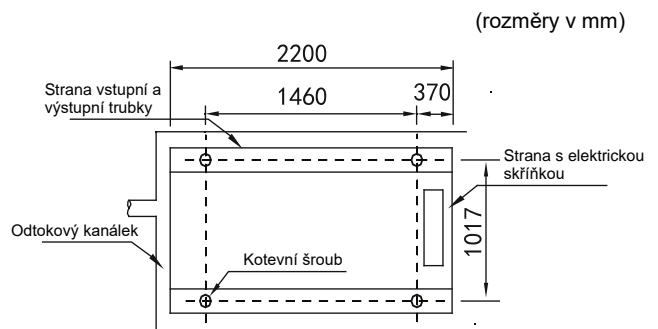
Obr. 6-7: Nákres instalačních rozměrů SCV-900EBH a SCV-1400EBH – pohled shora
