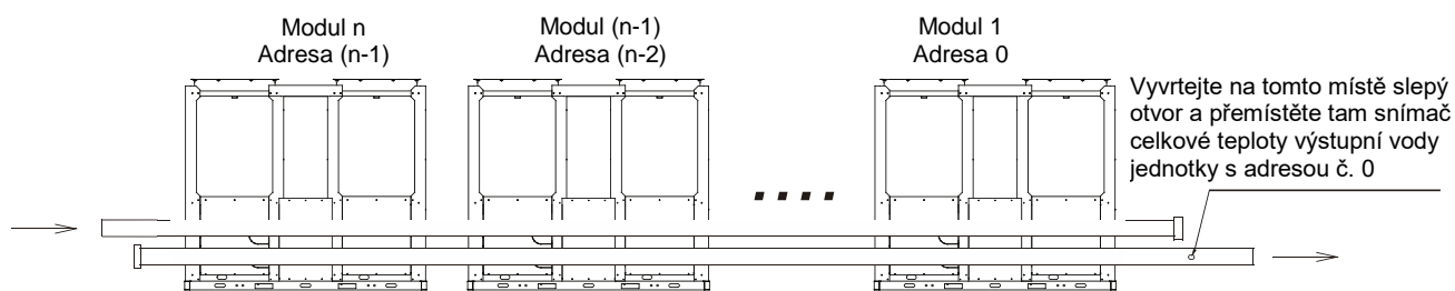
Obr. 8-32: Instalace několika modulů (max. 8 modulů) SCV-1800EBH
