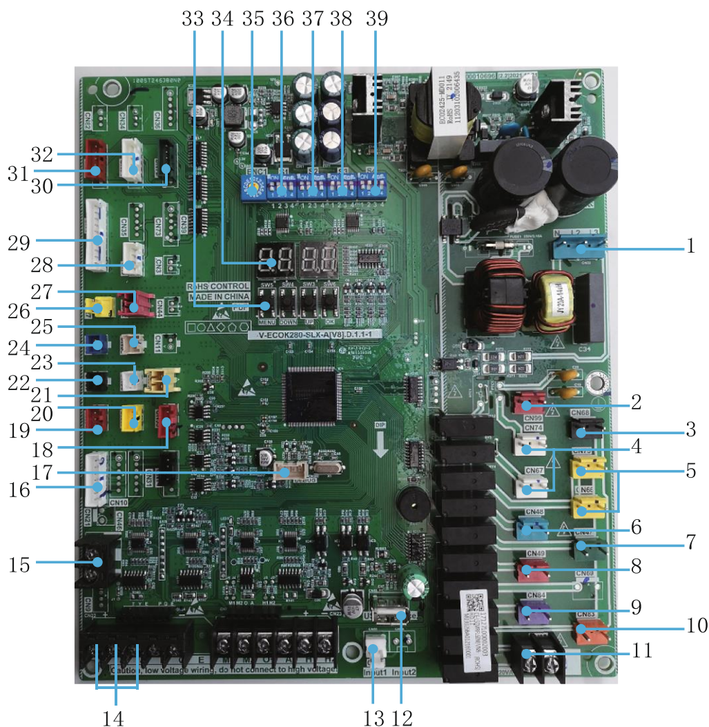
Obr. 8-9: Hlavní deska SCV-750EBH a SCV-1400EBH
