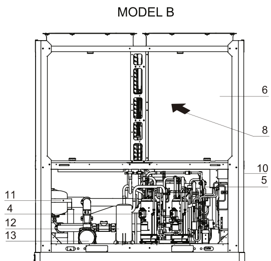
Obr. 8-4: Hlavní části SCV-1800EBH (Obrázek slouží jen pro zobrazení relativní pozice klíčových součástí)
