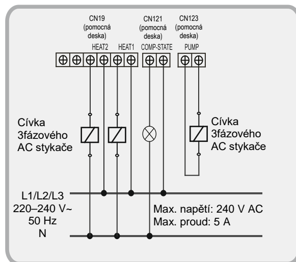
Obr. 8-19: Zapojení vodního čerpadla, pomocného ohřivače potrubí a AC kontrolky stavu kompresoru (pouze pro SCV-750EBH a SCV-1400EBH)
