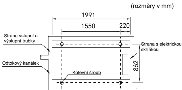
Obr. 6-6: Nákres instalačních rozměrů SCV-750EBH – pohled shora
