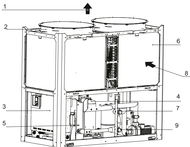
Obr. 8-1: Hlavní části SCV-750EBH (Obrázek slouží jen pro zobrazení relativní pozice klíčových součástí)
