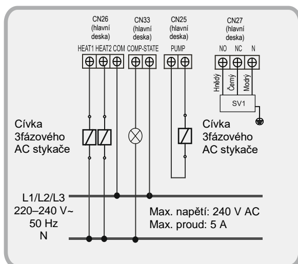
Obr. 8-20: Zapojení vodního čerpadla, pomocného ohřivače potrubí a AC kontrolky stavu kompresoru (pouze pro SCV-900EBH a SCV-1800EBH)
