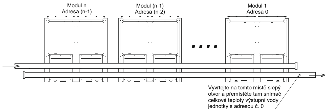
Obr. 8-31: Instalace několika modulů (max. 16 modulů)
