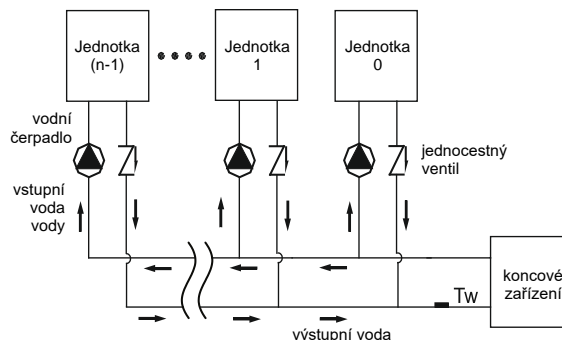
Obr. 8-34: Instalace několika vodních čerpadel
