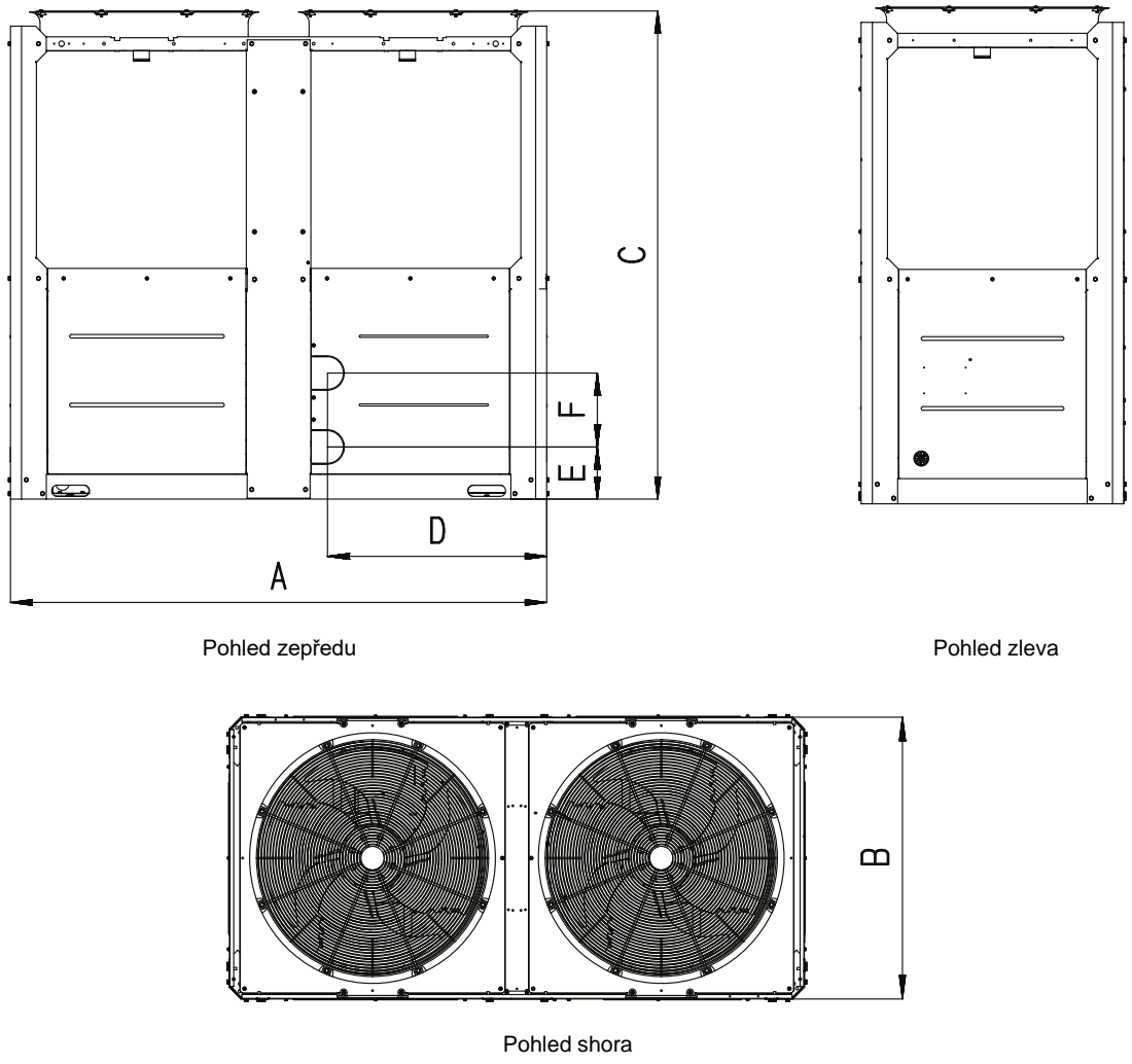
Obr. 6-1: Obrysové rozměry
