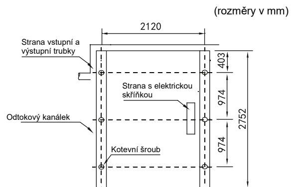
Obr. 6-8: Nákres instalačních rozměrů SCV-1800EBH – pohled shora
