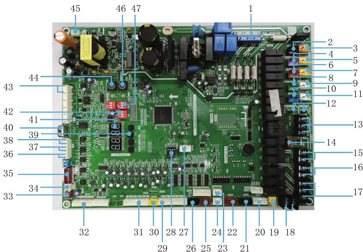
Obr. 8-11: Hlavní deska plošných spojů u SCV-900EBH a SCV-1800EBH
