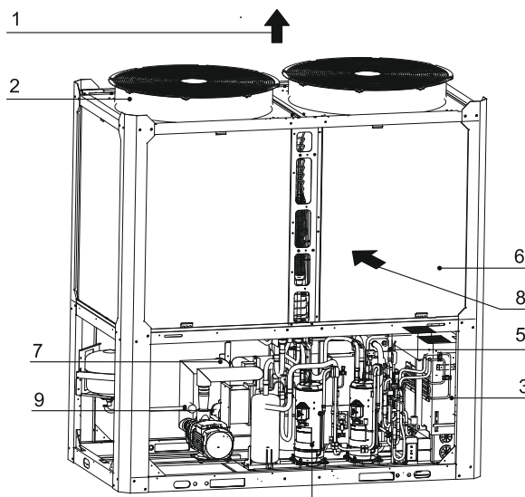
Obr. 8-2: Hlavní části SCV-900EBH (Obrázek slouží jen pro zobrazení relativní pozice klíčových součástí)
